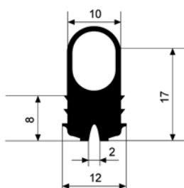
Referencia: 3213 Longitud rollo: 50 m. Material: EPDM 55° Negro
