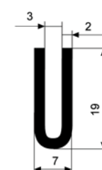
Perfil: 2203 Material: EPDM 65°
