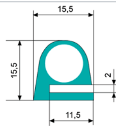
Referencia: S-123 Longitud rollo: 25 m. Material: MVQ Silicona-THT 60° Rojo oscuro
