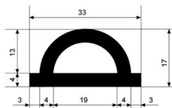
Referencia: 3439 Longitud rollo: 25 m. Material: Neopreno®/CR 55° Negro
