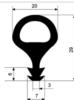
Referencia: 3143 Longitud rollo: 50 m. Material: EPDM 55° Negro
