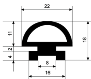
Referencia: 3453 Longitud rollo: 25 m. Material: Neopreno®/CR 55°
