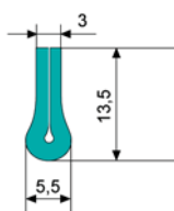
Referencia: S-111 Longitud rollo: 25 m. Material: MVQ Silicona-THT 60° Rojo oscuro
