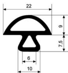
Referencia: 3220 Longitud rollo: 25 m. Material: EPDM 55° Negro
