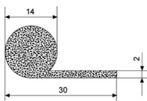
Referencia: PE597 Longitud rollo: 25 m. Material: NR esponjoso gris
