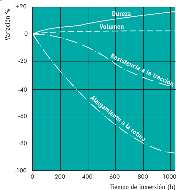
GRÁFICO 2. Variación de los valores característicos de los materiales (NBR) en función del tiempo de inmersión en aceites para engranajes SAE 80 a 100° C
