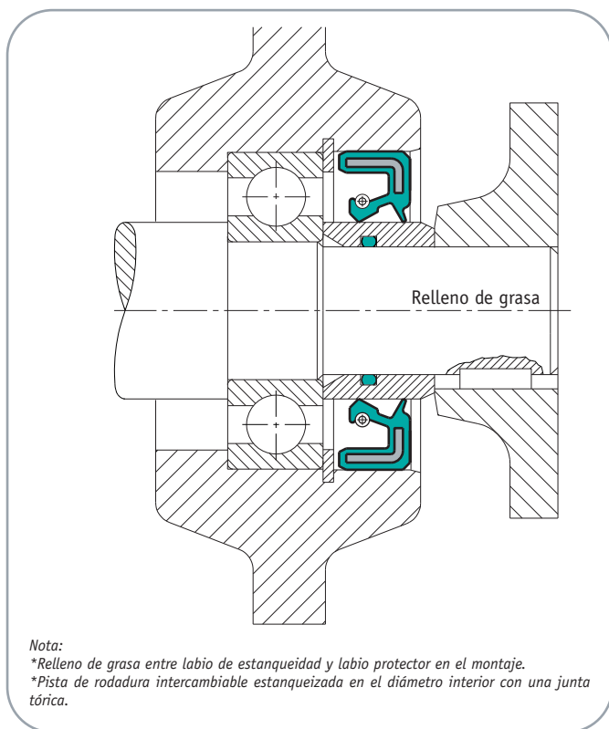
EJEMPLO DE MONTAJE 1: Estandarización de un rodamiento en caso de penetración de suciedad desde el exterior
