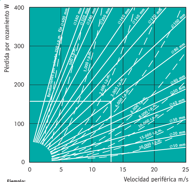
GRÁFICO 1. Pérdida por fricción en la estanqueización de aceites de motor SAE20 a 100° C con retenes radiales SIMMERRING®
