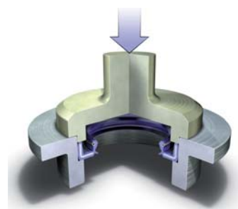
MONTAJE CON PRESA HIDRÁULICA O NEUMÁTICA
