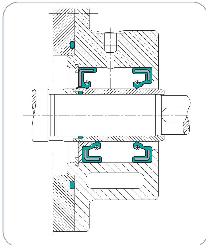
EJEMPLO DE MONTAJE 6: Obturación frente al vacío
