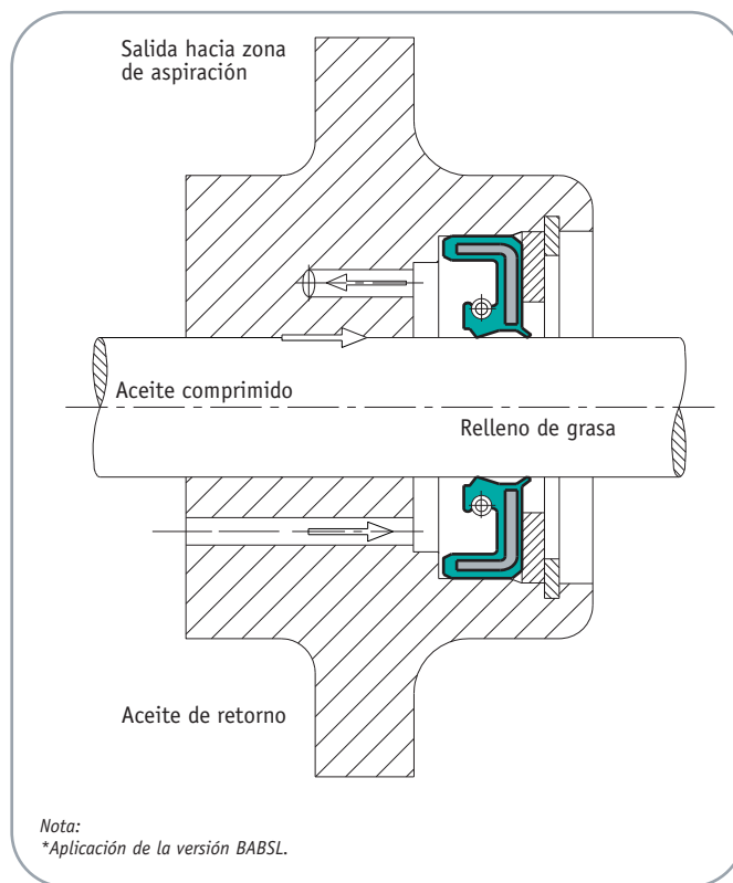
EJEMPLO DE MONTAJE 2: Estandarización bajo presión (ejemplo: bomba de aceite)
