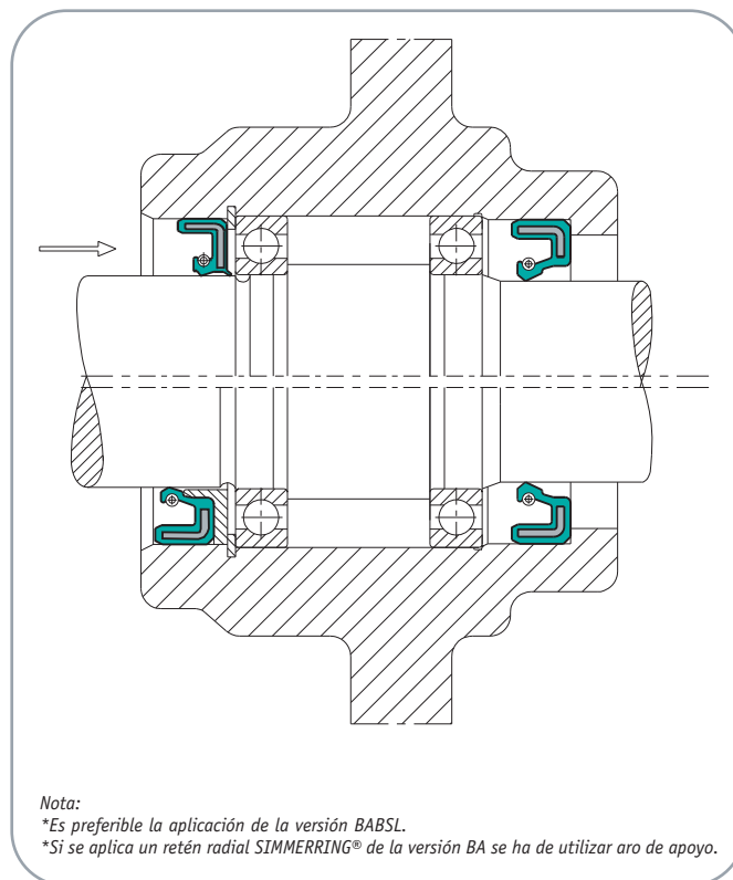
EJEMPLO DE MONTAJE 4: Obturación de aceite con baja presión
