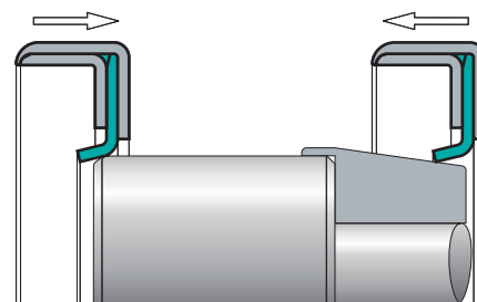
Montaje de un reten radial SIMMERRING® con labio de estanqueidad de PTFE
