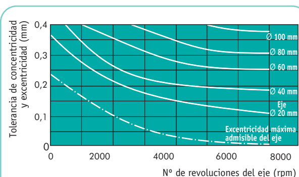
GRÁFICO 11. Tolerancia de concentricidad y excentricidad dinámica en función del número de revoluciones para la versión BASL
