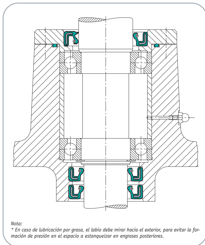
EJEMPLO DE MONTAJE 8: Obturación de un eje vertical
