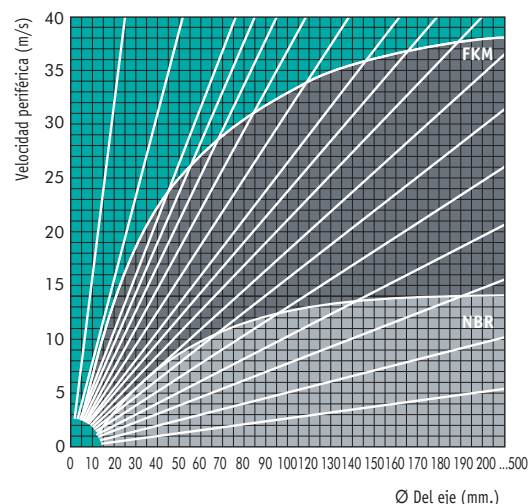
GRÁFICO 5. Velocidades periféricas admisibles para retenes radiales SIMMERRING® en los materiales 72 NBR 902 y 75 FPM 585, para la estanqueización de aceite para motores SAE 20.
