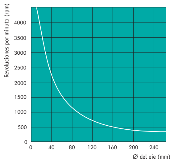
GRÁFICO 8. Número de revoluciones admisible para retenes radiales SIMMERRING® en rotación
