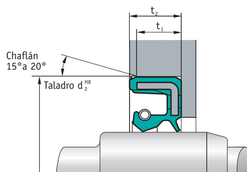
Dimensiones de los chaflanes y alojamientos
