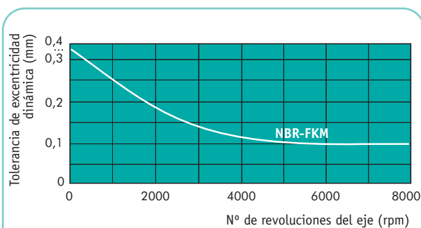
GRÁFICO 10. Tolerancia máxima de la excentricidad dinámica del eje en función del número de revoluciones
