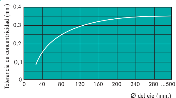
GRÁFICO 9. Tolerancia máxima de la concentricidad en función del diámetro del eje
