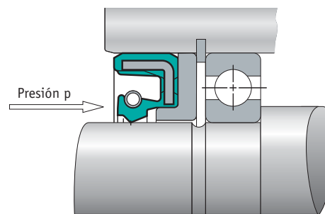
Instalación de un retén SIMMERRING® con anillo de apoyo
