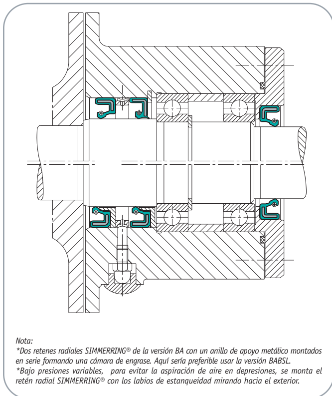
EJEMPLO DE MONTAJE 5: Obturación de agua a presión ligera
