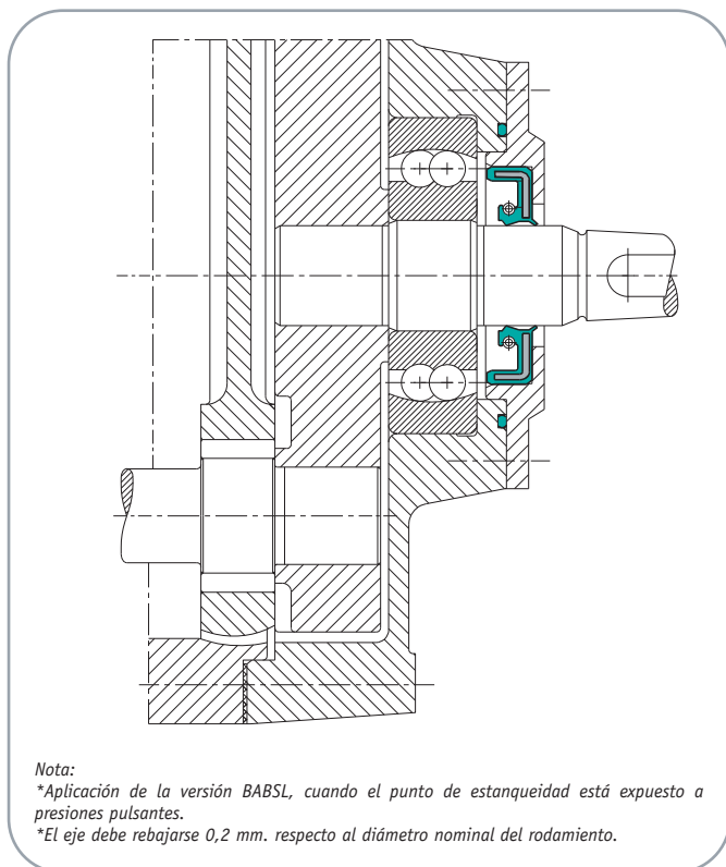
EJEMPLO DE MONTAJE 3: Estandarización bajo presión (ejemplo: cigüeñal de un motor de dos cilindros)
